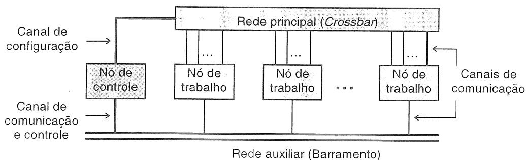
Figura 1: Arquitetura do multicomputador Crux.
