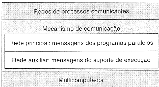
Figura 2: Mecanismo de comunicação com atribuição de canais físicos por demanda.
